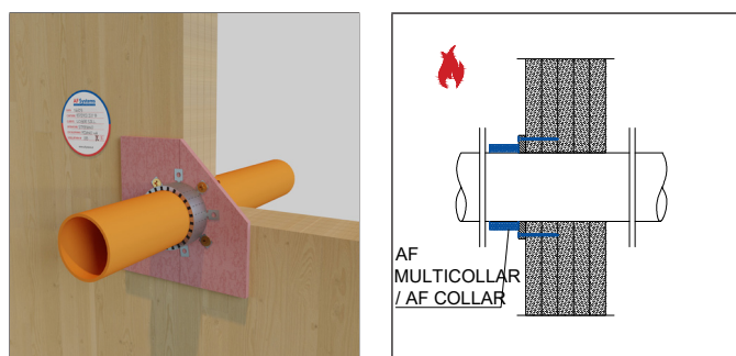
Parete Xlam
