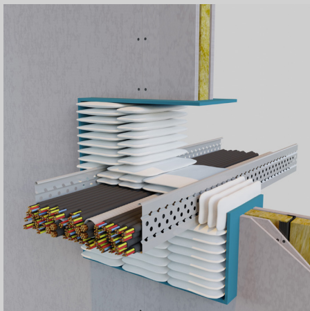
Figura 4b | Profondità di sigillatura 320 mm
