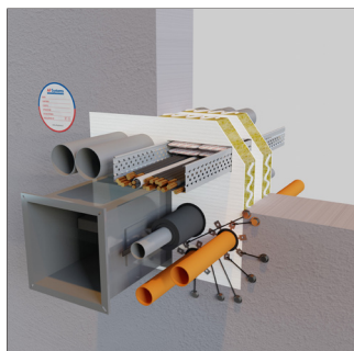
Parete Rigida
