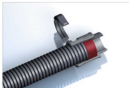
PMAFIX, IP68
